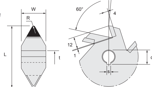
Пазовая фреза
